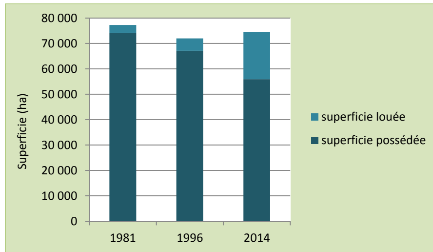
Figure 17 – Superficies des terres exploitées et en location dans la MRC des Appalaches pour les années 1981, 1996 et 2014 d'après les données du MAPAQ
